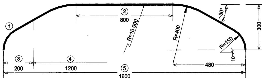
Фигура 3.1 Профил на колекторна глава на токоснемател
