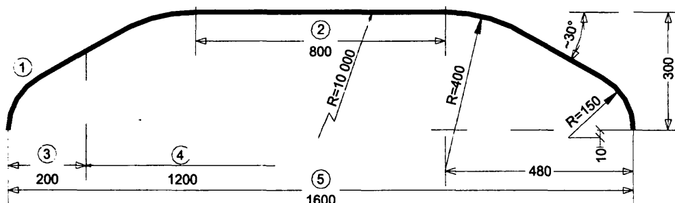
Фигура 4.1 Профил на колекторната глава на токоснемателя
