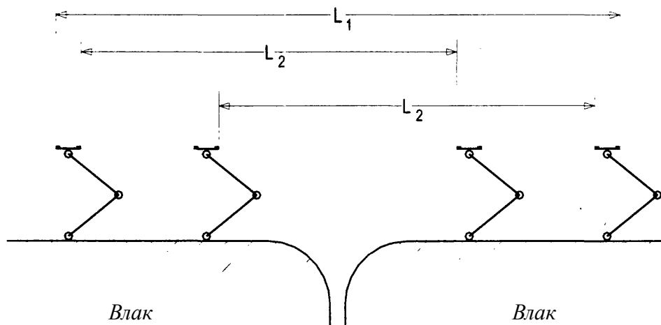
Фигура 3.5 Подреждане на токоснематели
