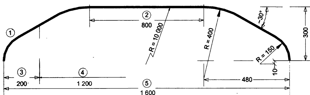
Фигура Й.1 Профил на колекторната глава на токоснемател
