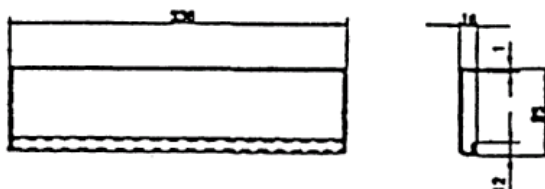
Фигура 3 Пример за корито за събиране на течността (размерите са в милиметри)
